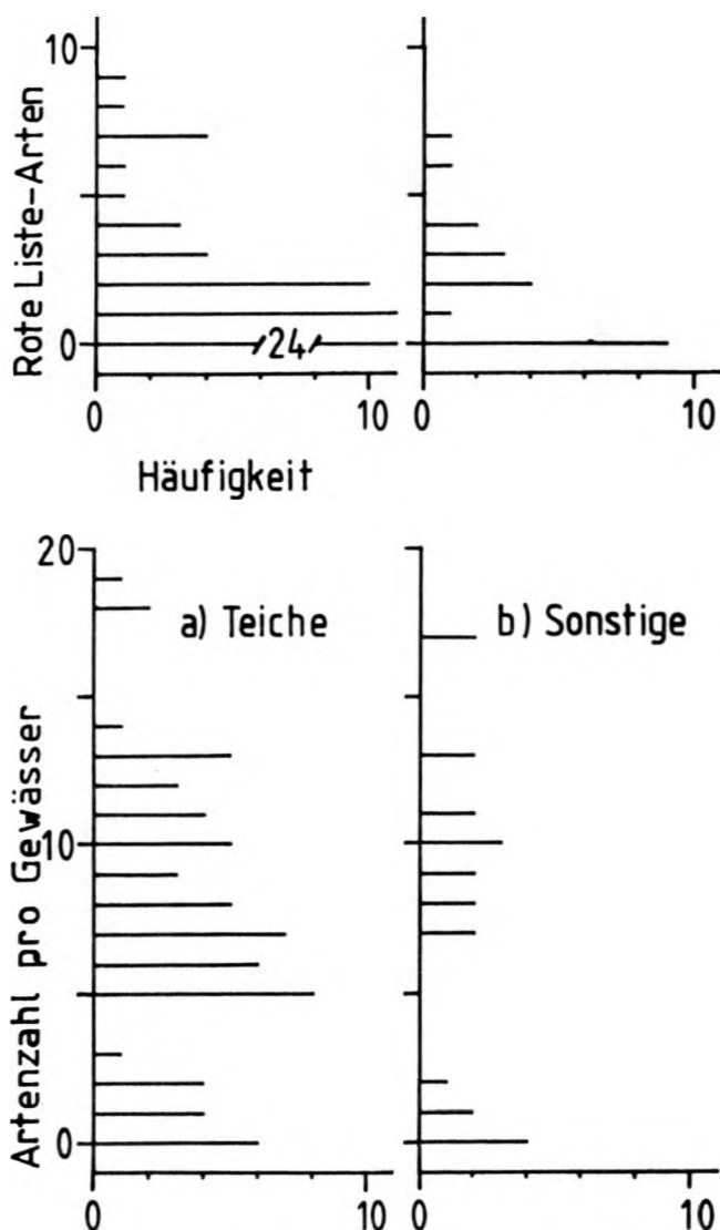
Abb. 3: Verteilung der Gesamtartenzahl und der Anzahl Rote-Liste-Arten pro Gewässer, aufgetrennt nach Gewässertyp:
