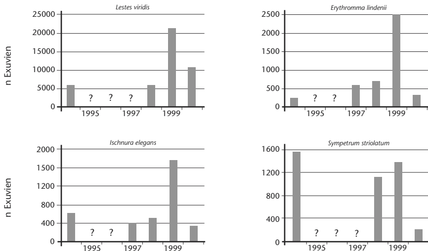
Abbildung 5: Emergenzraten 1994 bis 2000 von Lestes viridis , Erythromma lindenii , Ischnura elegans und Sympetrum striolatum an der Hexenkehle. — Figure 5: Emergence rates from 1994 to 2000 of Lestes viridis , Erythromma lindenii , Ischnura elegans and Sympetrum striolatum at the 'Hexenkehle' (Baden-Wuerttemberg, Germany).
