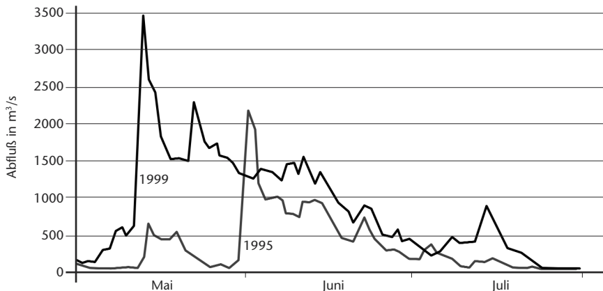
Abbildung 1: Abflüsse des Restrheins (Pegel Rheinweiler) während der Monate Mai, Juni und Juli der Jahre 1995 (grau) und 1999 (schwarz). Quelle: Wasser- und Schifffahrtsamt Freiburg. — Figure 1: Discharge of the river "Restrhein" (water gauge Rheinweiler; Baden-Wuerttemberg, Germany) during May, June, and July of the years 1995 (grey) and 1999 (black).
